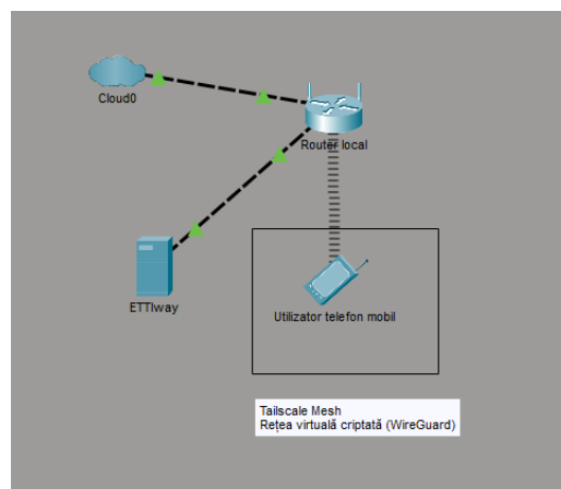
Figura 3.4: Topologia rețelei platformei ETTIway.
